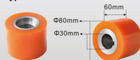
PU款 U0303 PU Type
