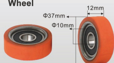
自动封边机轮 U0602 Automatic Edge Bander Wheel
