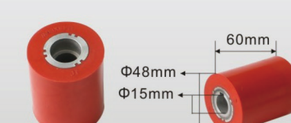
通用款 U0406 Universal Type
