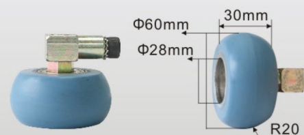
巴贝兰 U0501 Bauberan Type
