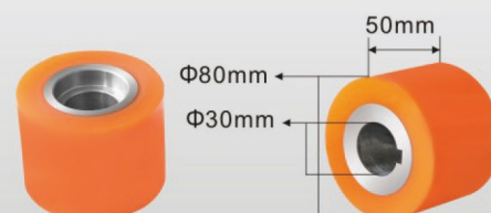
PU款 U0302 PU Type
