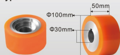
PU款 U04004 PU Type
