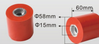
通用款 U0407 Universal Type
