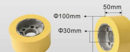
通用款 U0405 Universal Type
