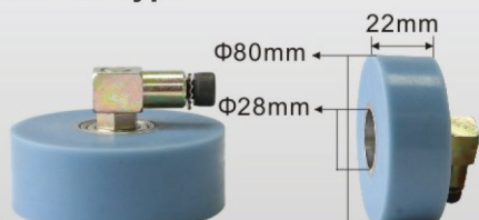
巴贝兰 U504 Bauberan Type
