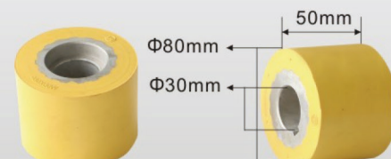
橡胶款 U0406L Rubber Type
