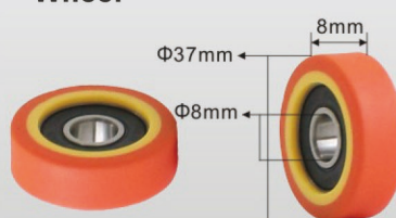
自动封边机轮 U0606 Automatic Edge Bander Wheel
