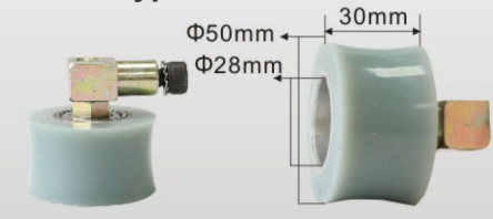
巴贝兰 U0503 Bauberan Type
