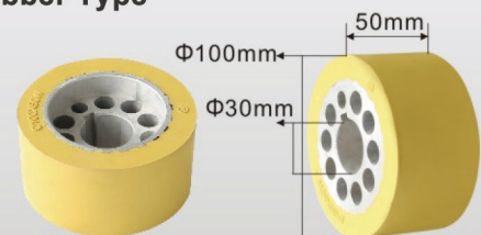
橡胶款 U0407L Rubber Type
