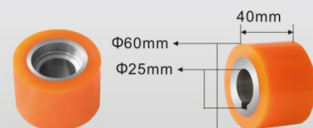
PU款 U0301 PU Type
