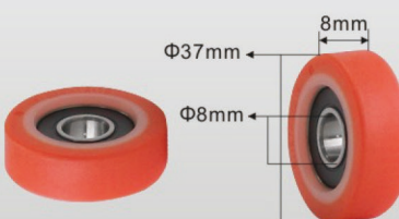
自动封边机轮 U0605 Automatic Edge Bander Wheel
