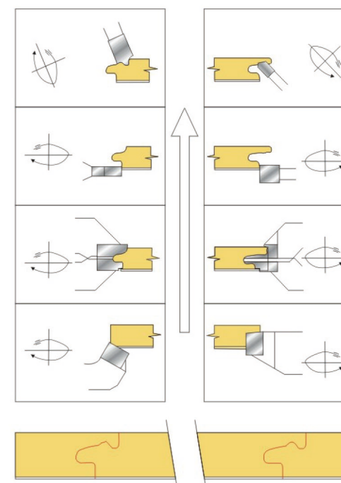
硬质合金地板刀
