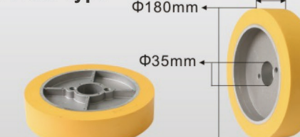
通用款 U0404 Universal Type
